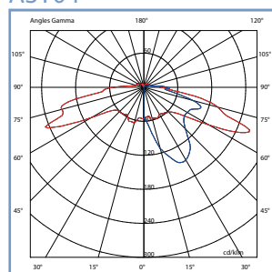
Courbes polaire / Polar curves
